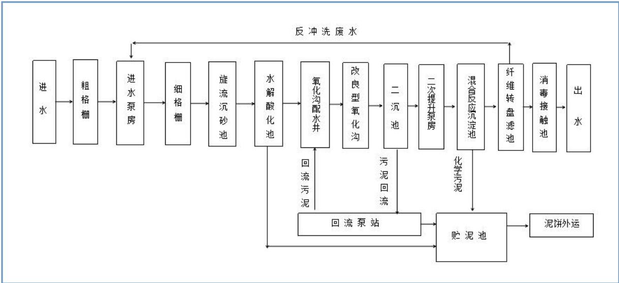
主体工艺流程图：
