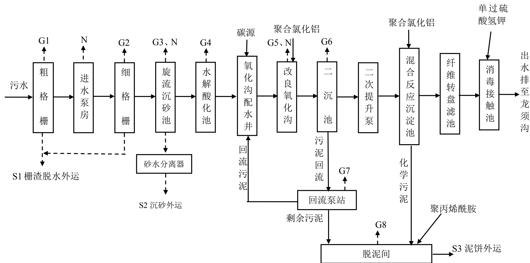
图 2-2 污水处理厂二期工程污水处理工艺
